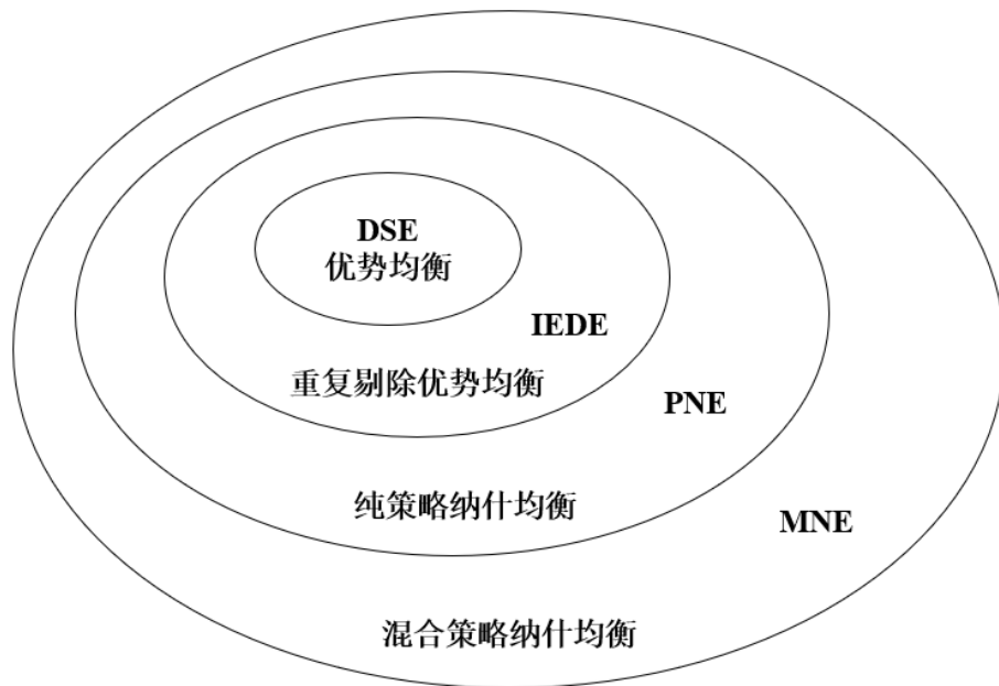
图 1.6 不同均衡概念之间的关系
